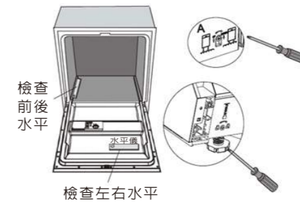
【圖8】腳調整圖示 註：腳的最大調整行程是50mm
