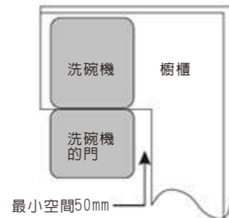
【圖2】 門打開時最小空間
